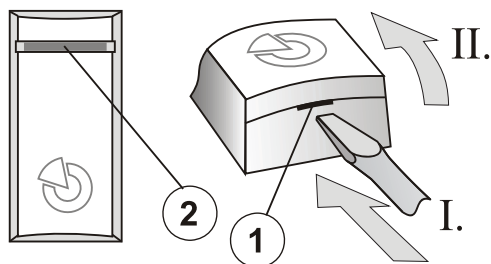
Рис: 1 – защелка крышки; 2 – светодиоды (желтый и красный)
